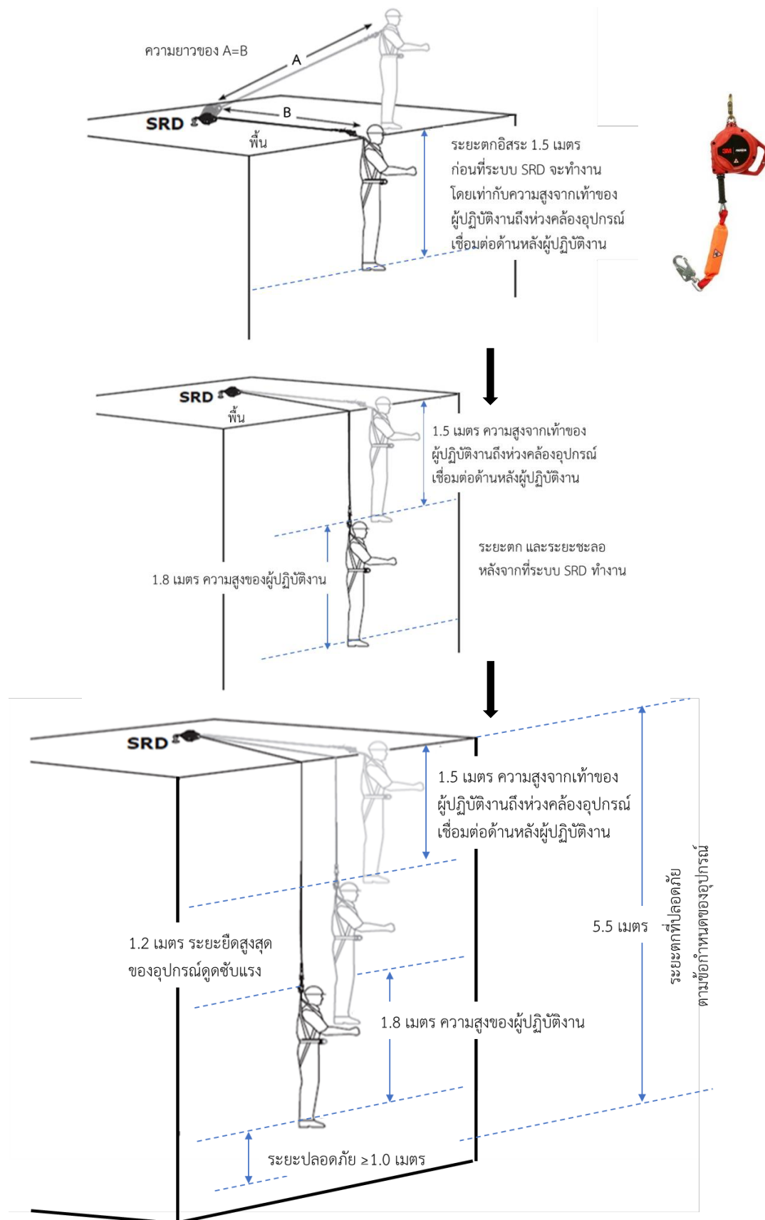
ภาพที่ 2-32 การคำนวณระยะการตกที่ปลอดภัยของเชือกนิรภัยชนิดดึงกลับอัตโนมัติแนวราบ
