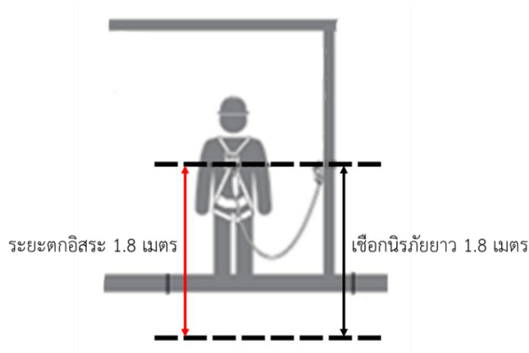
ภาพที่ 2-36 จุดยึดเกี่ยวเสมอตำแหน่งจุดคล้องเกี่ยว
