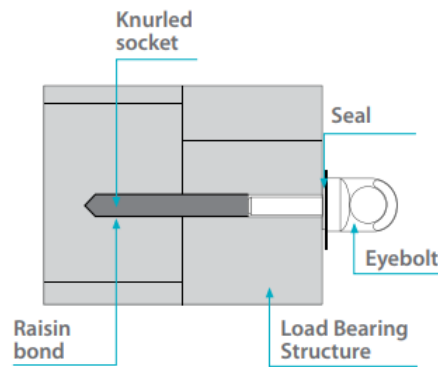
ภาพที่ 2-6 ตัวอย่างจุดยึดเกี่ยวเคมีคัลลี บอนด์
