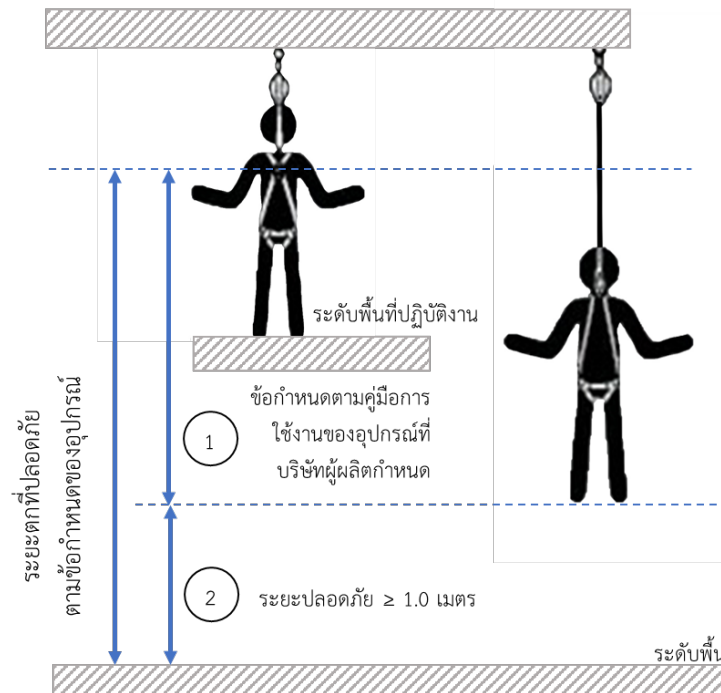
ภาพที่ 2-31 การคำนวณระยะการตกที่ปลอดภัยของเชือกนิรภัยชนิดดึงกลับอัตโนมัติแนวดิ่ง
