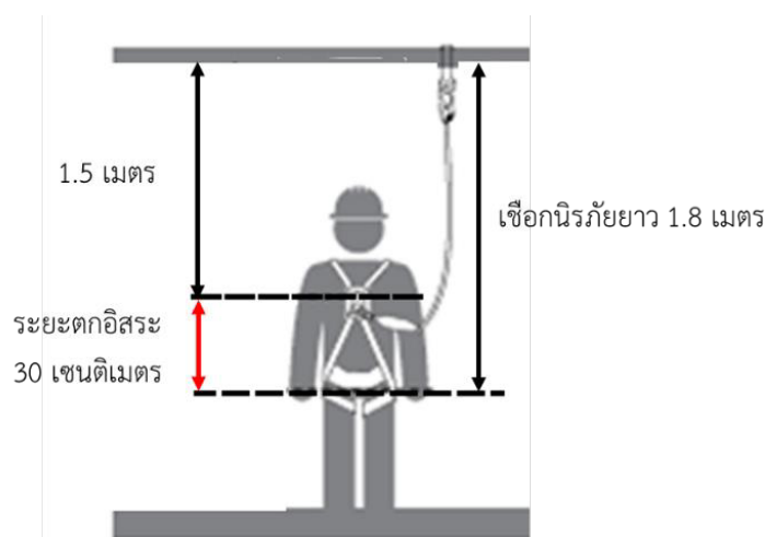
ภาพที่ 2-35 จุดยึดเกี่ยวสูงกว่าจุดคล้องเกี่ยว
