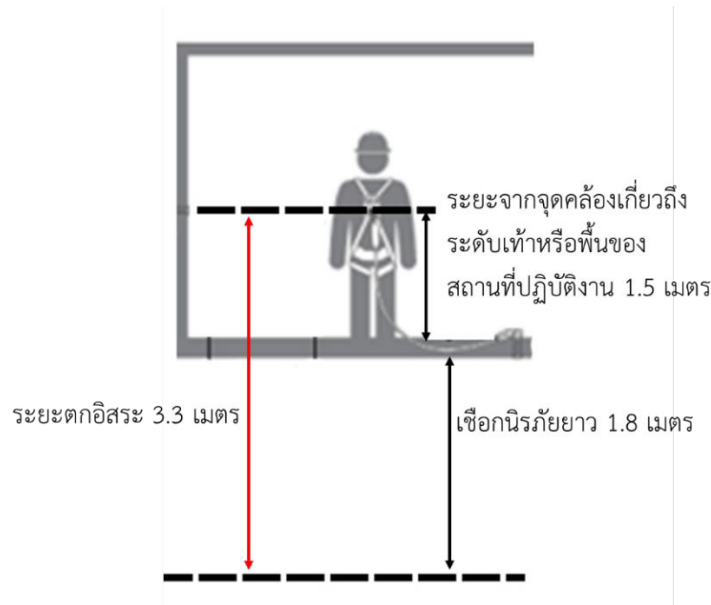
ภาพที่ 2-37 จุดยึดเกี่ยวต่ำกว่าตำแหน่งจุดคล้องเกี่ยว
