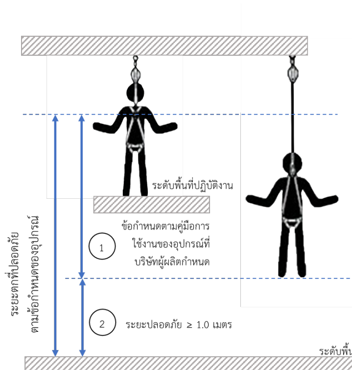
ภาพที่ 2-31 การคำนวณระยะการตกที่ปลอดภัยของเชือกนิรภัยชนิดดึงกลับอัตโนมัติแนวดิ่ง
