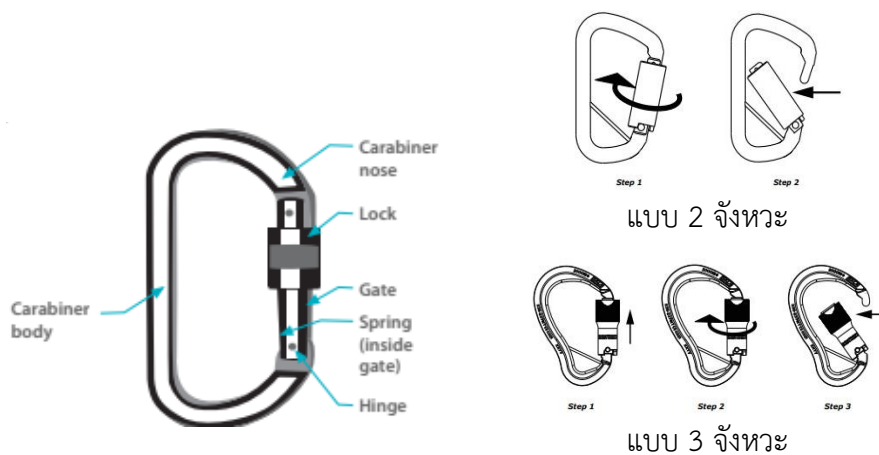
ภาพที่ 2-12 ตัวอย่างห่วงเกี่ยวนิรภัยชนิดคาราไบเนอร์
