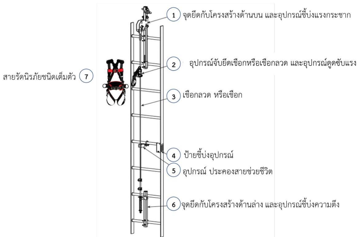
ภาพที่ 2-29 สายช่วยชีวิตที่ออกแบบติดตั้งแบบถาวรในแนวดิ่ง
